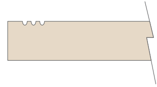
●踏板断面図 (すべり止め3本R溝加工)
