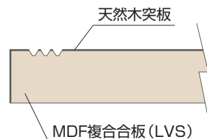
●踏板断面図 (すべり止め3本V溝加工)
