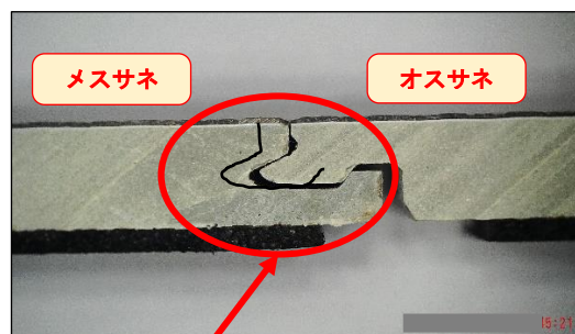
(長辺側のサネ嵌合の断面)
