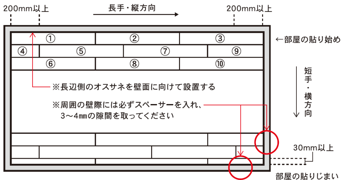
[割付図 1]
